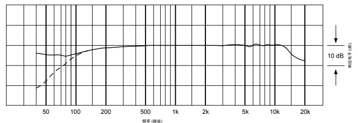
电平 —— 平直 - - - - 高通滤波 (MTS30a)
