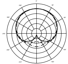
声压曲线1刻度5 dB 频率 200 Hz 1 kHz 5 kHz 8 kHz
